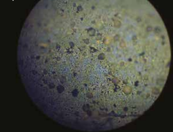
VISTA AL MICROSCOPIO A RIFLESSIONE UV DI UNA MESCOLA BITUME POLIMERO CONTENENTE MICROSFERE DI VETRO PURISSIMO
