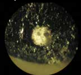
VISTA AL MICROSCOPIO A RIFLESSIONE UV DI UNA MESCOLA BITUME POLIMERO CONTENENTE MICROSFERE DI VETRO PURISSIMO
