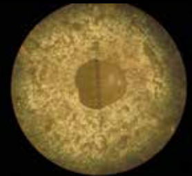
VISTA AL MICROSCOPIO A RIFLESSIONE UV ED AL MICROSCOPIO OTTICO DI UNA MESCOLA BITUME POLIMERO CONTENENTE MICROSFERE DA ROTTAMI DI VETRO
