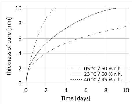
Diagramma 1: Velocità di vulcanizzazione Sikasil® WS-200
