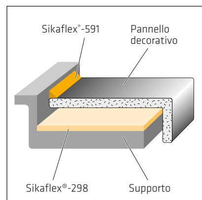
Incollaggio verticale di un pannello decorativo
