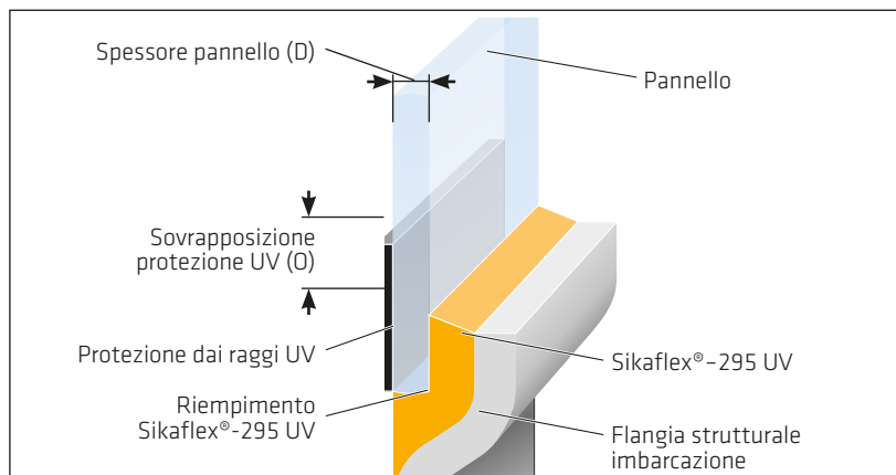
Incollaggio verticale di un pannello decorativo
