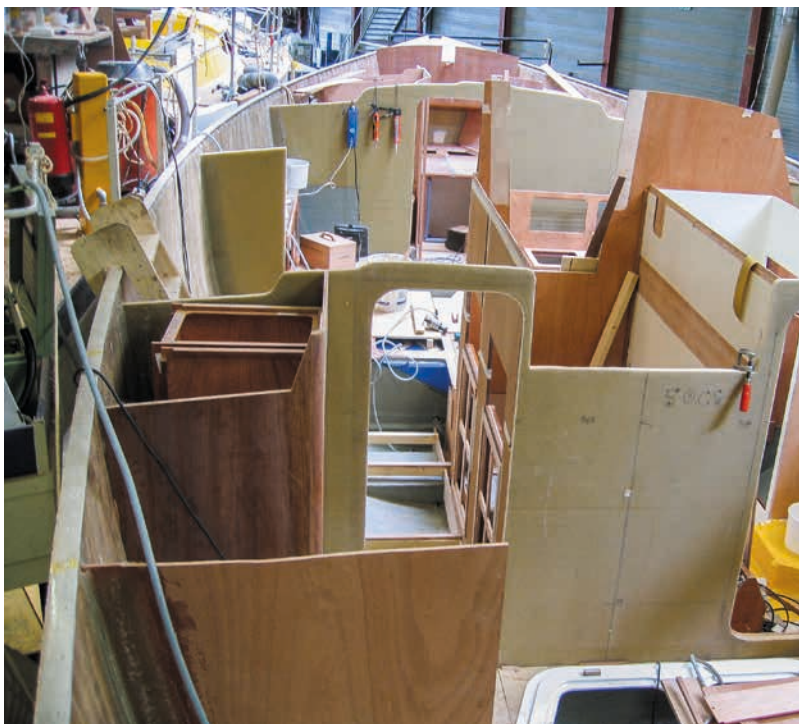
Pannelli leggeri montati su uno scafo aperto
