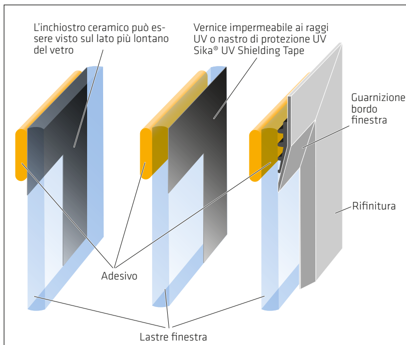
Incollaggio verticale di un pannello decorativo
