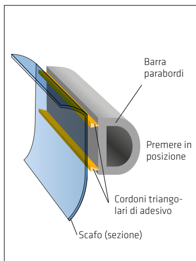
Assemblaggio di barra parabordi
