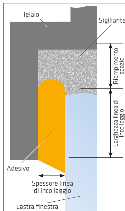
Incollaggio verticale di un pannello decorativo
