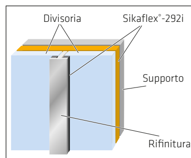
Applicazione di cordone di Sikaflex®-292i per l'incollaggio del supporto
