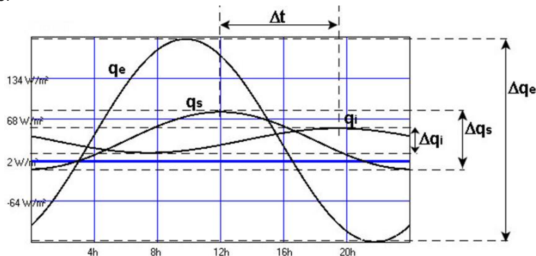
Figura 3.5 Distribuzione della temperatura e del flusso nell'arco di 24 ore. I grafici mostrano l'andamento dei parametri per una parete soggetta a una sollecitazione climatica sinusoidale sul lato esterno.
