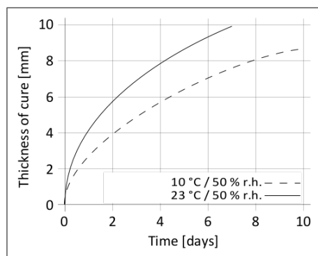
Figura 1: Velocità di indurimento di SikaTack® MAX 30 (Purform®)
