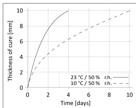
Grafico 1: Velocità polimerizzazione SikaTack® TRANSPORT (Purform®)
