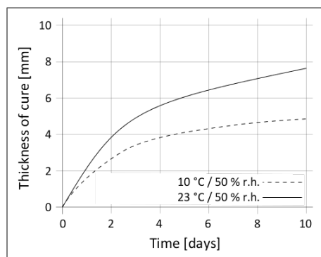
Grafico 1: Velocità di indurimento Sikaflex®-529 Evolution
